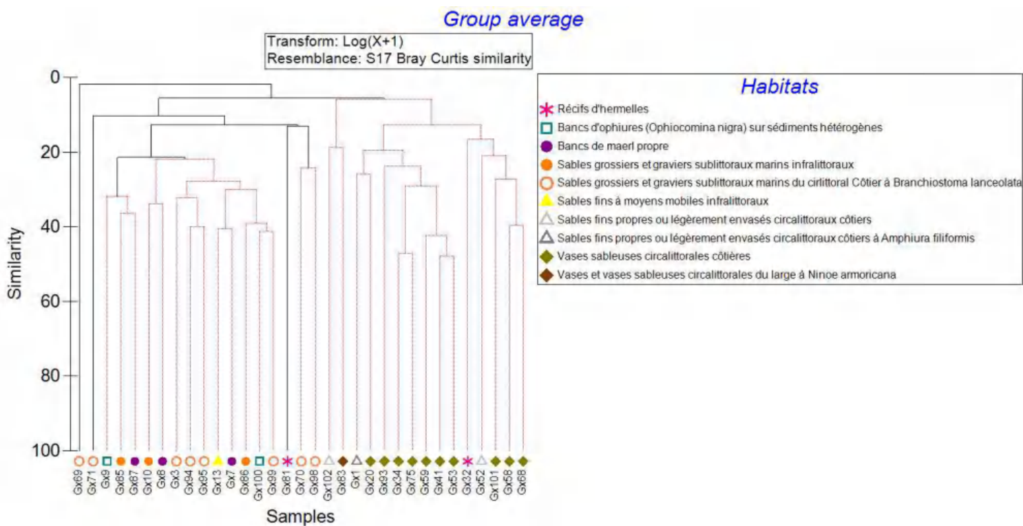
Figure 47: Dendrogramme sur la matrice faune des dragues Rallier du Baty sur les données transformées en \text{Log}(X+1) .
