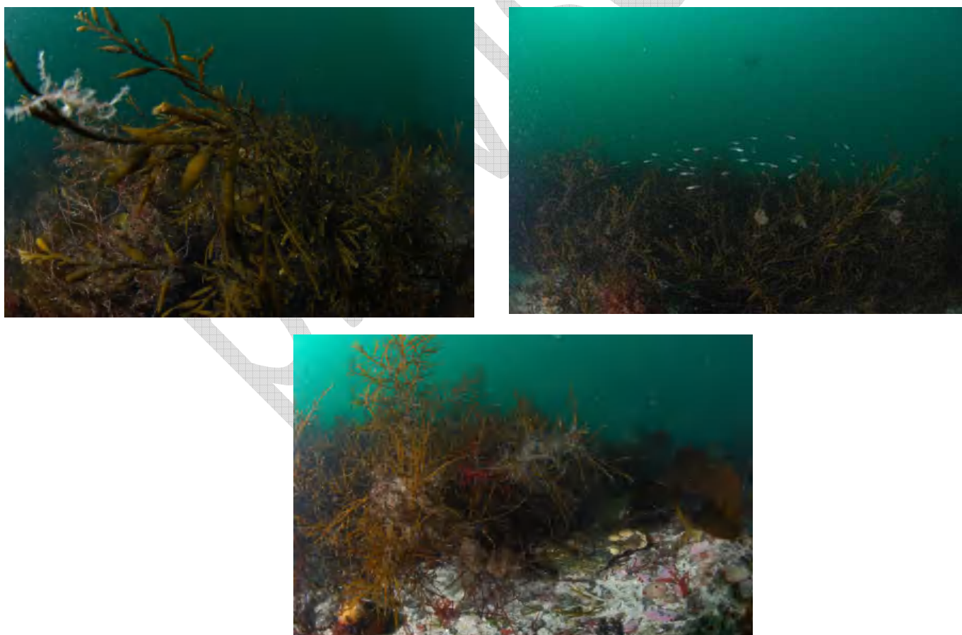
Figure 36: Habitat Ceinture infralittorale à Halidrys siliquosa sur Groix (Clichés TBM-LEMAR)
